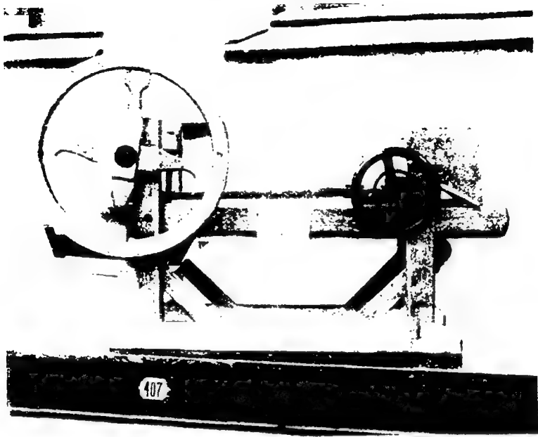
Рис. 2. Трещетка Бломериуса.
